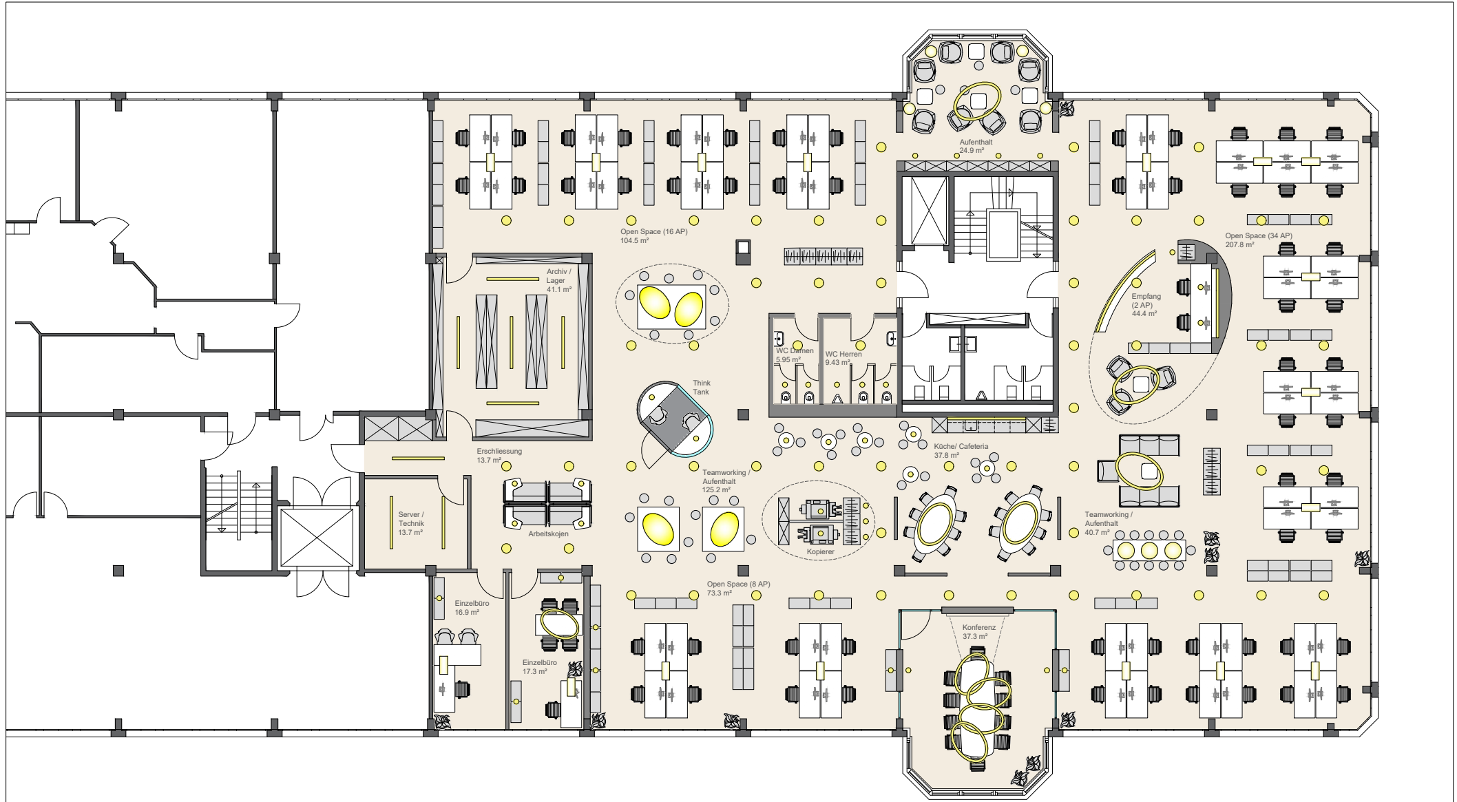
5507 Blegistr Baar - Beleuchtungskonzept - 1.Obergeschoss - Büroraum 01-0101 (04_201218)
